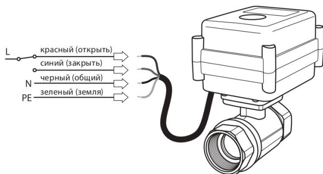
Рис. 1 Электрическая схема подключения крана с электроприводом серии Neptun AquaControl 220B
