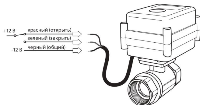
Рис. 2 Электрическая схема подключения крана с электроприводом серии Neptun AquaControl 12B
