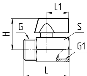
Рисунок 2 – Габаритные размеры крана.
