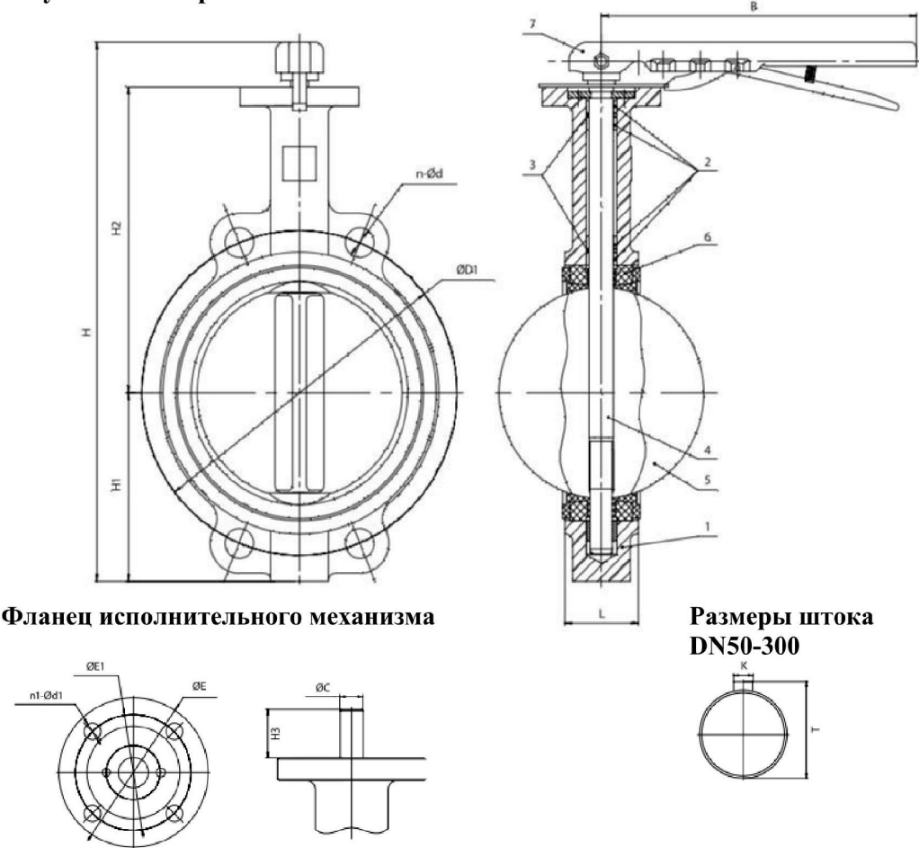
Рисунок 1. Затворы DN 50-300
