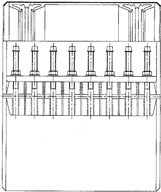
Наружный ремонтный хомут
