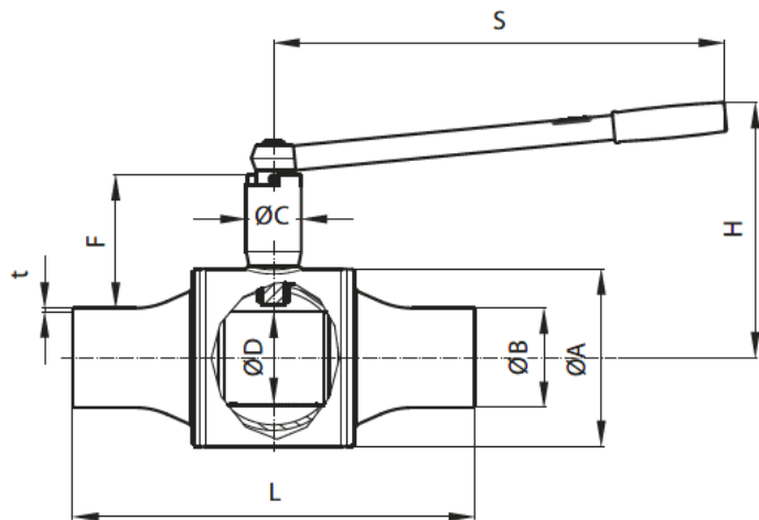
Габаритные и присоединительные размеры кранов шаровых типа JiP Full Borec патрубками под приварку.
