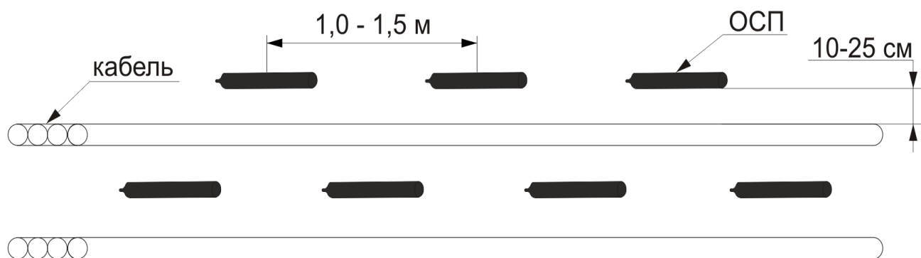
Рисунок 2 - Пример размещения ОСП для защиты горизонтальных кабельных трасс
