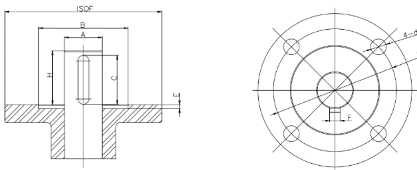
Рис. 3. Фланец под редуктор.
