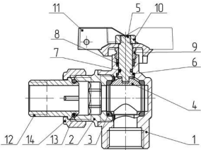
Рисунок 1 – Конструкция шарового крана
