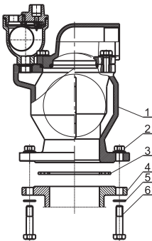
Схема монтажа
