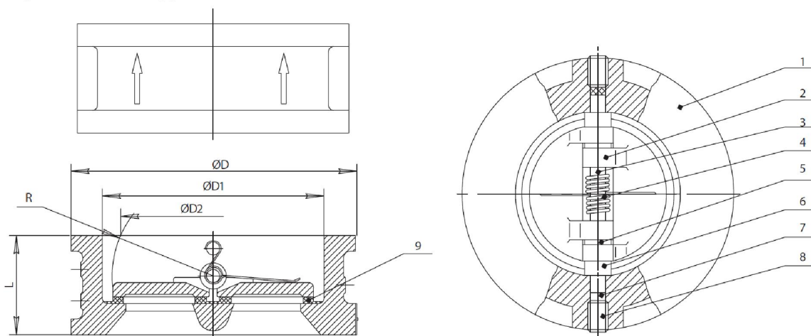
Рисунок 1. Конструкция клапана
