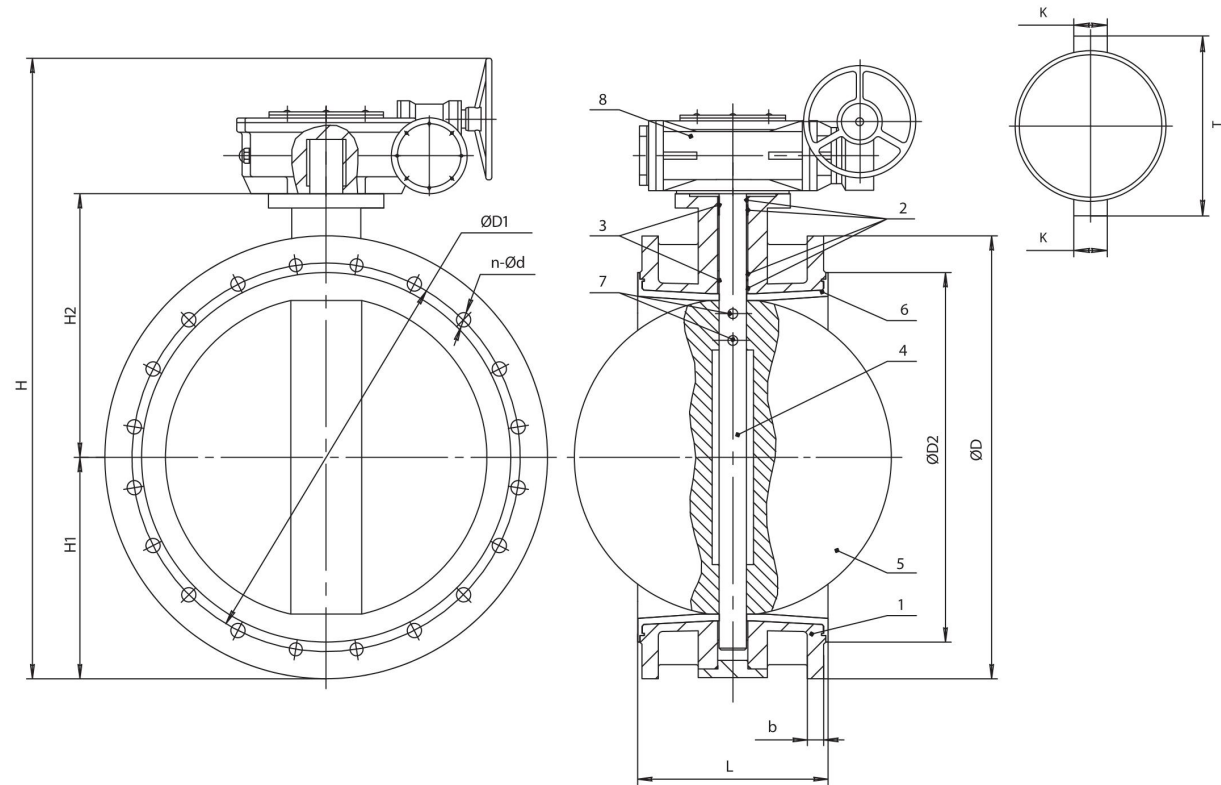
Рисунок 2. Затворы с редуктором DN 350-1400
