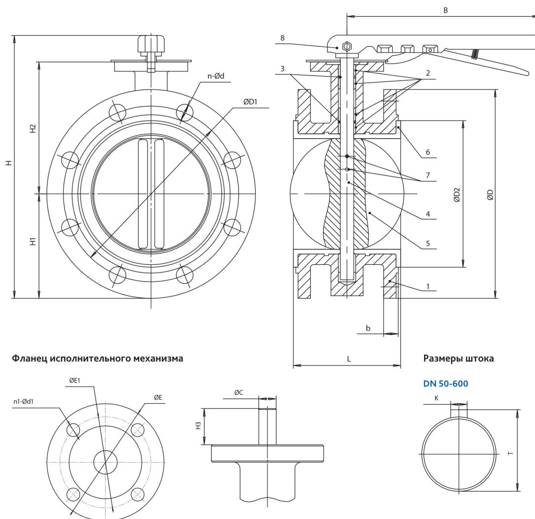
Рисунок 1. Затворы с рукояткой DN 50-300
