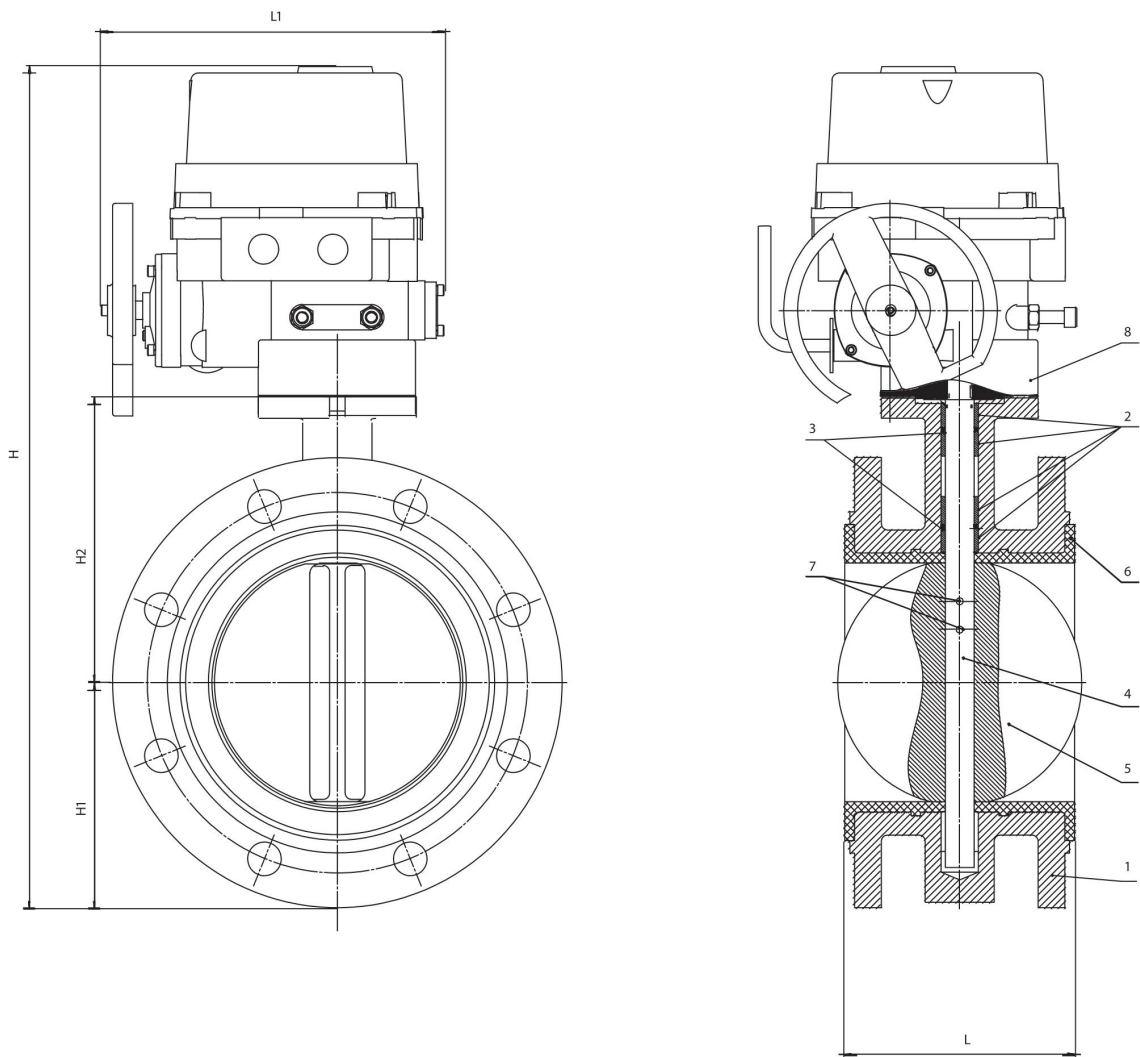
Рисунок 3. Затворы с электроприводом DN 50-300
