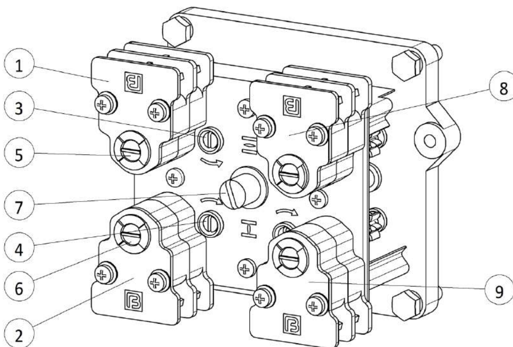
Рисунок 14 – Ограничитель хода с путевыми выключателями
