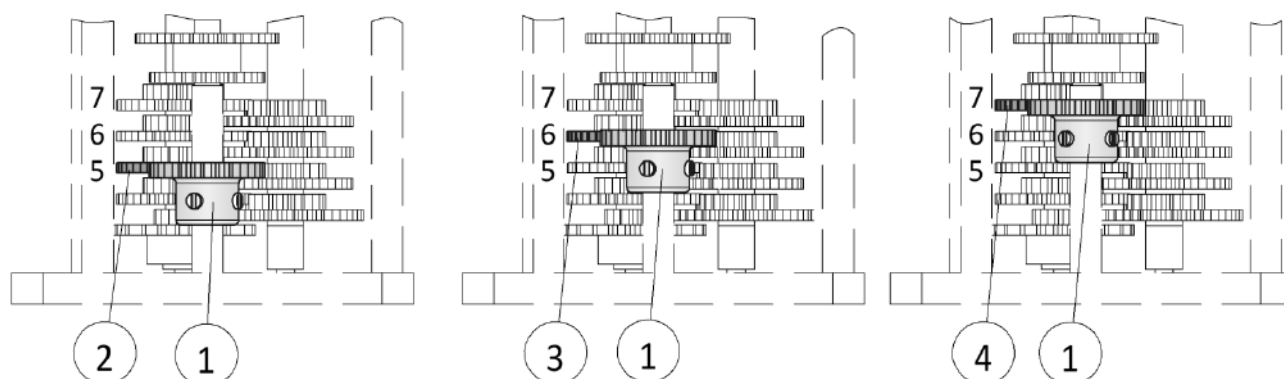
Рисунок 10 – Настройка диапазона рабочего хода указателя
