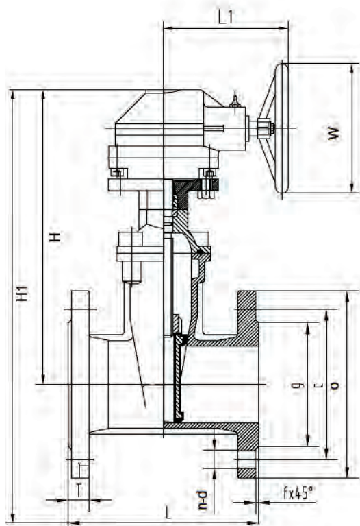
Чертеж габаритный задвижки клиновой с обрезиненным клином и невыемным штоком ABRA-A40-16XXXG DN 40-300 чугунной ABRA-A40-10XXXG DN 200-300 чугунной (размеры в таблице ниже)
