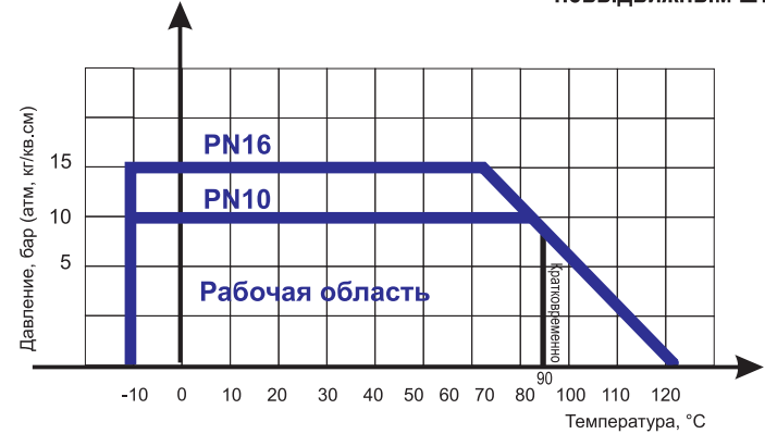
Диаграмма Давление / Температура для задвижки клиновой ABRA-A40-10-XXXG и ABRA-A40-16-XXXG с обрезиненным клином и невыеданным штоком DN 40-1000, PN 10 и PN 16
