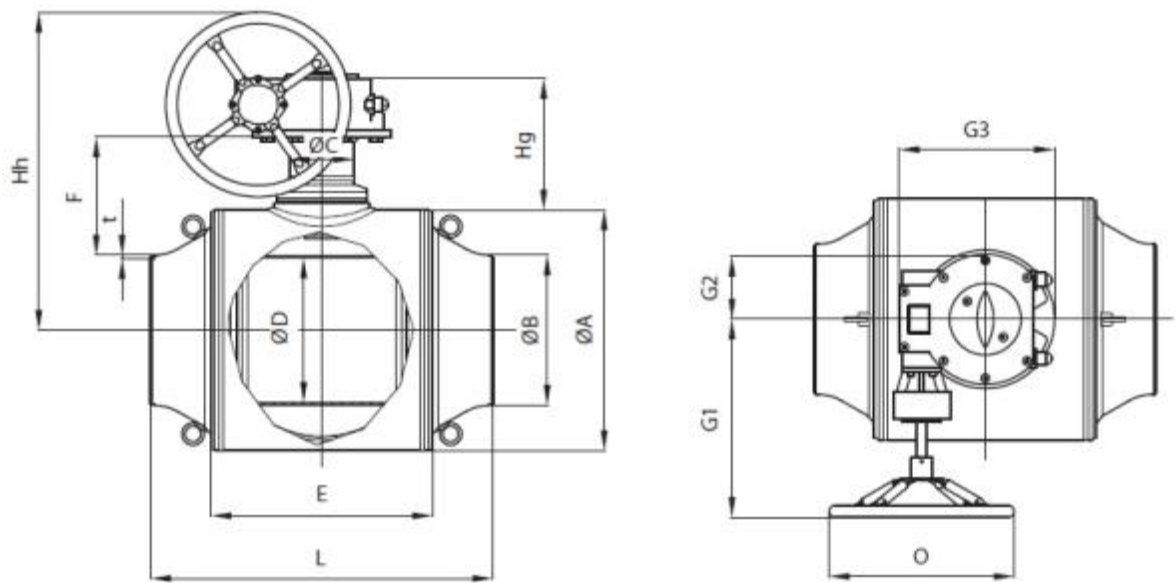
Габаритные и присоединительные размеры кранов шаровых типа JIP с рукояткой и патрубками под приварку.
