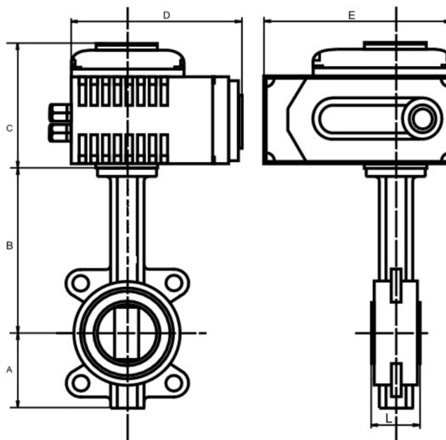
Чертеж габаритный затвора поворотного ABRA BUV-VF с электроприводом Сатурн, DN 32-DN 300
