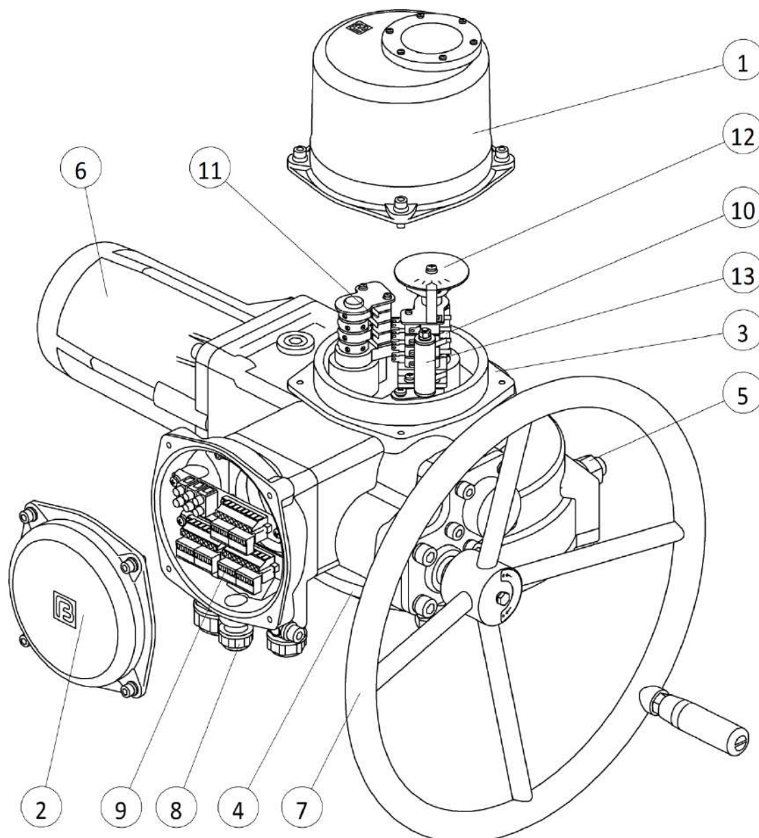
Рисунок 1 – Общий вид электропривода
