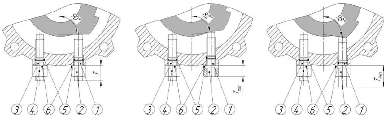
Рисунок 5 – Концевые упоры
