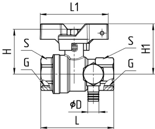
Рисунок 2 – Габаритные размеры крана.
