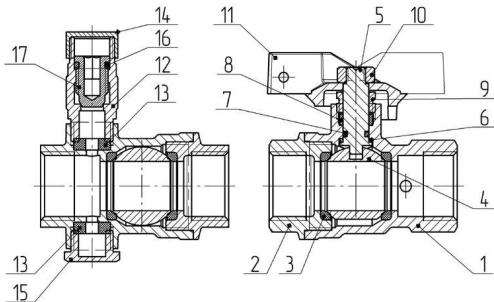
Рисунок 1 – Конструкция шарового крана со спускником
