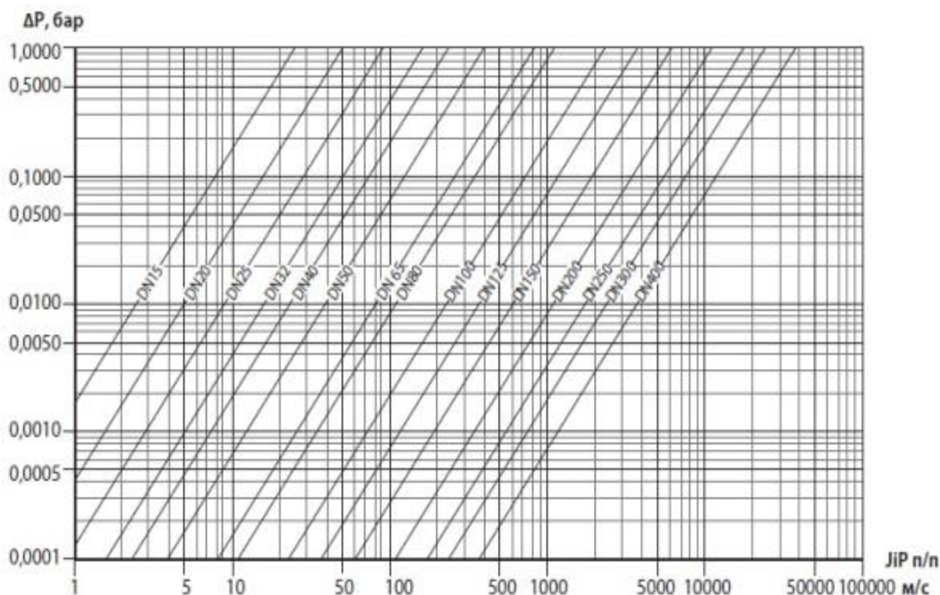
Диаграмма потерь давления крана шарового типа JiP Full Bore.
