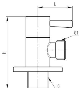
Рисунок 2 – Габаритные размеры клапана (вентиля).
