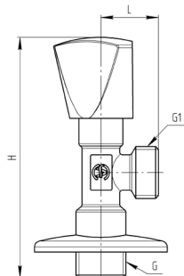
Рисунок 2 – Габаритные размеры клапана (вентиля).
