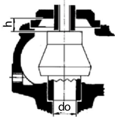
Высота подъема седла h
