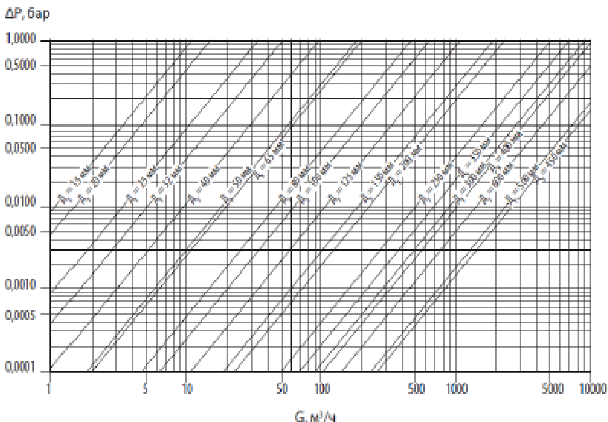
Диаграмма потерь давления крана шарового модификации JiP Premium
