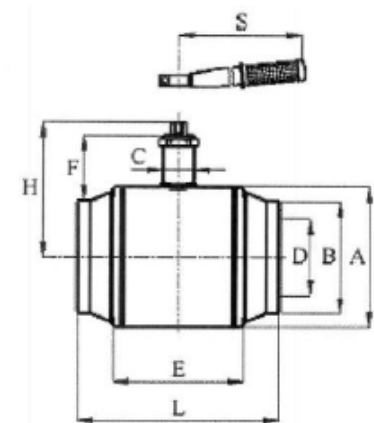
Габаритные и присоединительные размеры кранов шаровых типа JiP с рукояткой и патрубками под приварку.
