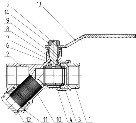
Рисунок 1 – Конструкция шарового крана
