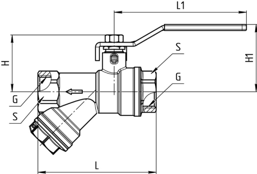
Рисунок 2 – Габаритные размеры крана.
