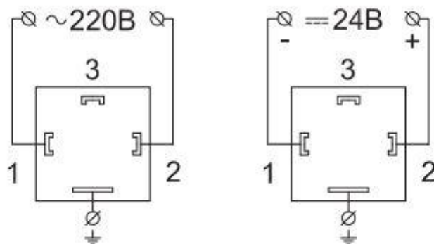
Схемы подключения катушки
