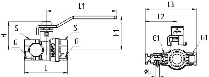
Рисунок 2 – Габаритные размеры крана.
