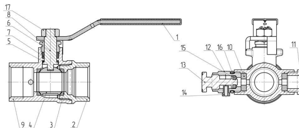
Рисунок 1 – Конструкция шарового крана
