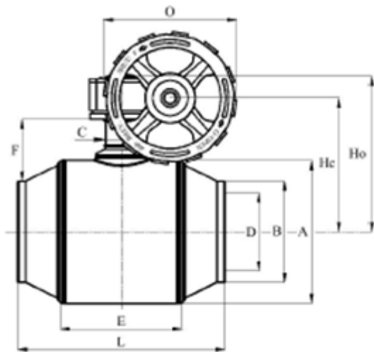
Габаритные и присоединительные размеры кранов шаровых типа J1P с рукояткой и патрубками под приварку.
