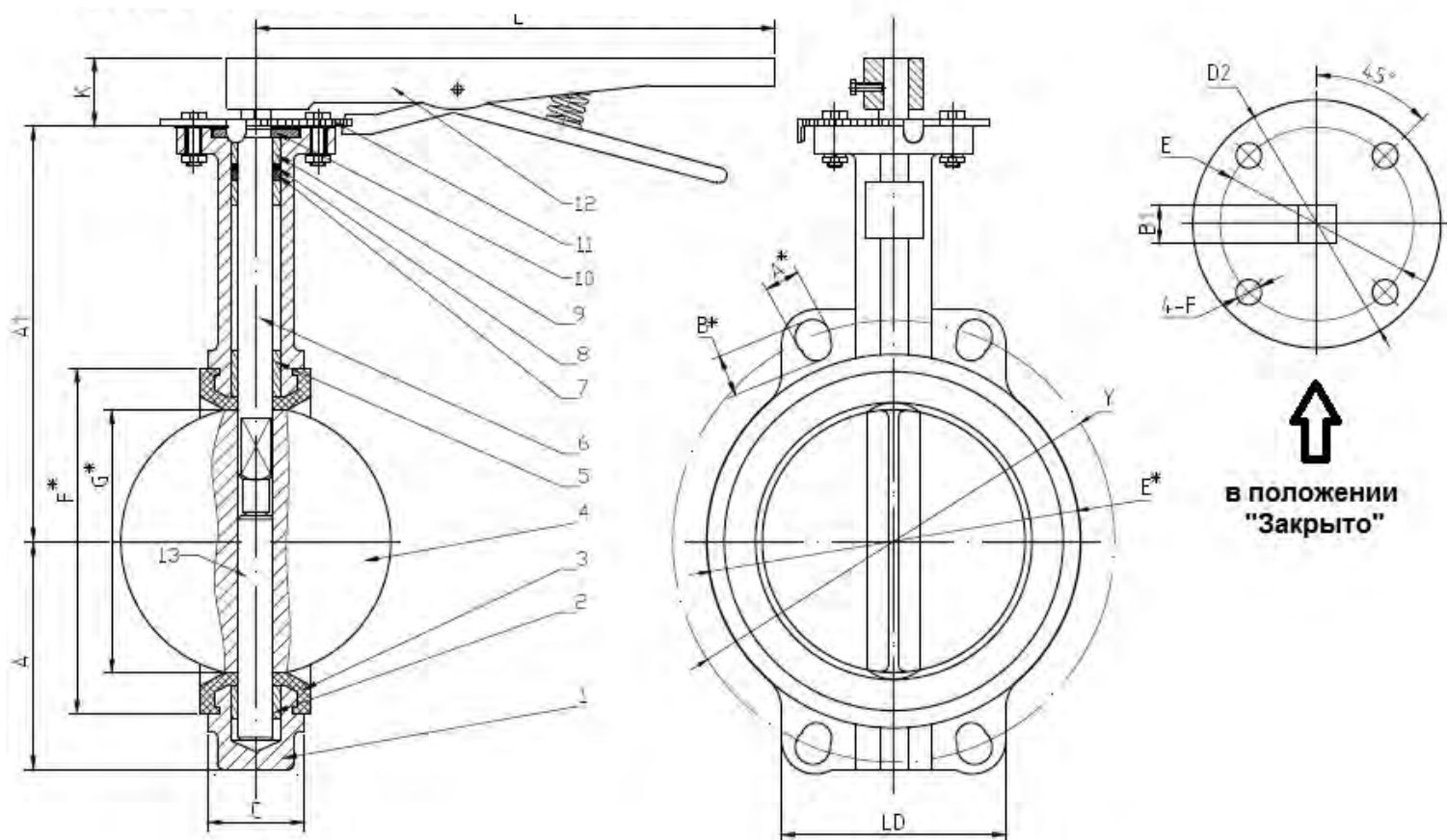
ABRA-BUV-VF863 DN100-300 PN10/16
