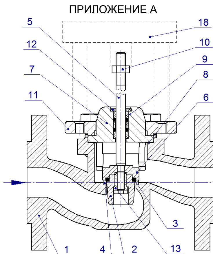
Рисунок А.1 Устройство неразгруженного по давлению клапана DN 15 ÷ DN 32
