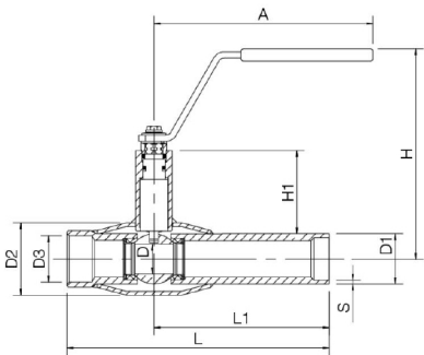
DN 10-50
