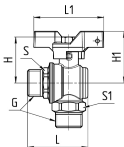
Рисунок 2 – Габаритные размеры крана.
