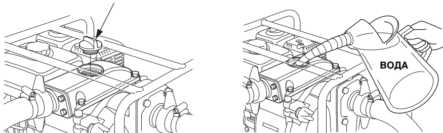
ПРОБКА ГОРЛОВИНЫ ВОДЫ ДЛЯ ПРЕДВАРИТЕЛЬНОЙ ПРОКАЧКИ
