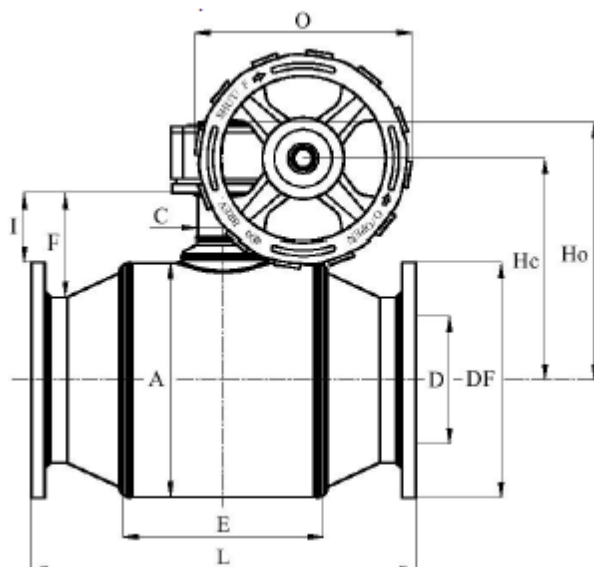
Габаритные и присоединительные размеры кранов шаровых типа JiP, фланцевые.
