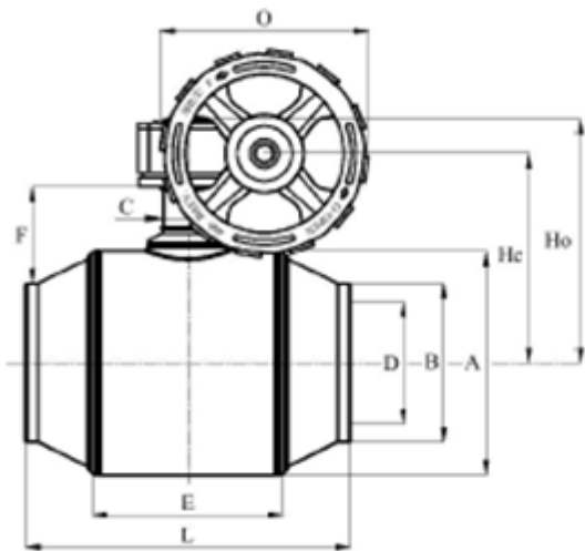
Габаритные и присоединительные размеры кранов шаровых типа JiP с рукояткой и патрубками под приварку.
