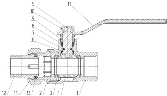
Рисунок 1 – Конструкция шарового крана
