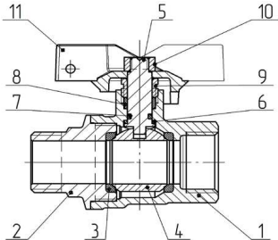
Рисунок 1 – Конструкция шарового крана
