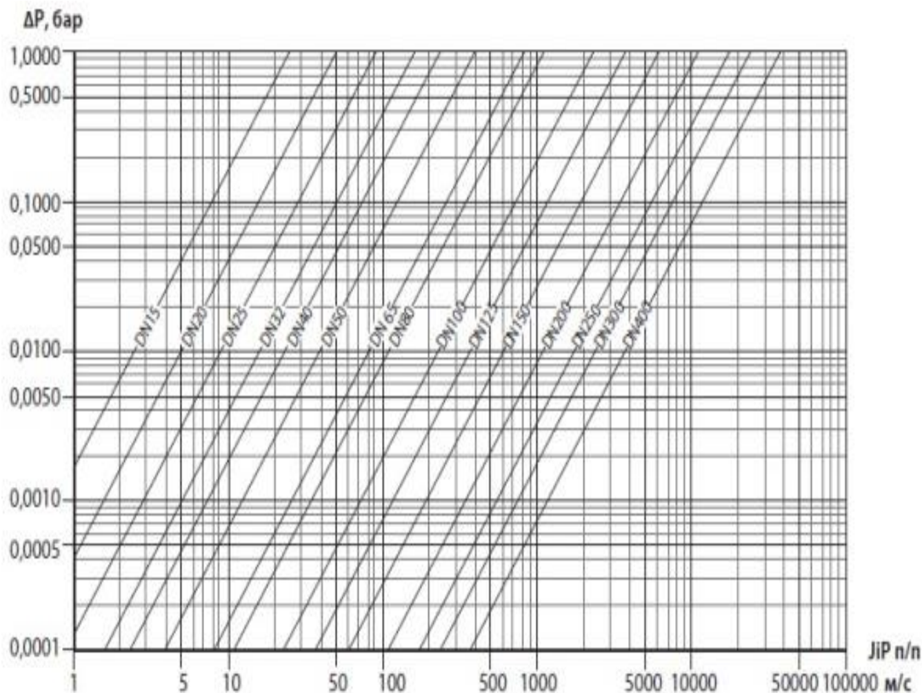
Диаграмма потерь давления крана шарового типа JIP Full Bore.
