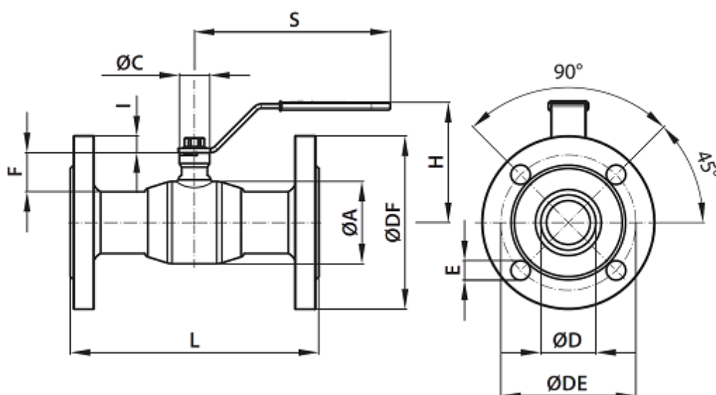
Габаритные и присоединительные размеры кранов шаровых типа RJIP, фланцевые.
