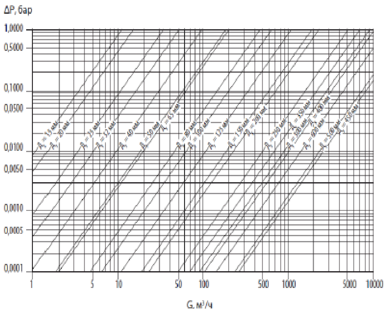
Диаграмма потерь давления крана шарового модификации JiP Premium
