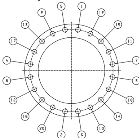
Рис. 1 Схема затяжки болтов
