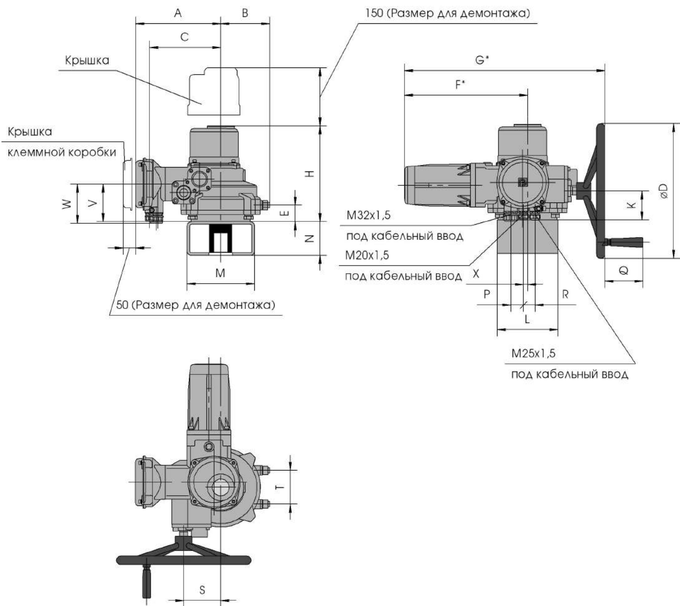
Размеры в миллиметрах
