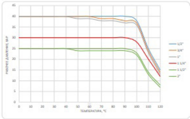
График 1 – Зависимость давления от температуры
