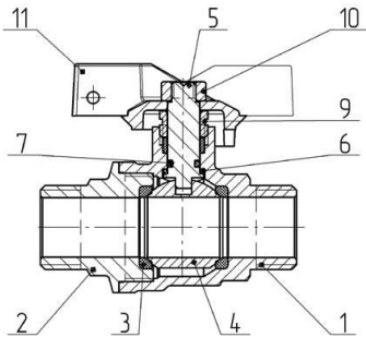
Рисунок 1 – Конструкция шарового крана
