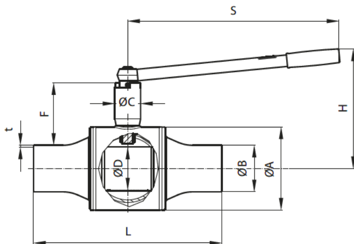
Габаритные и присоединительные размеры кранов шаровых типа JiP Full Borec патрубками под приварку.
