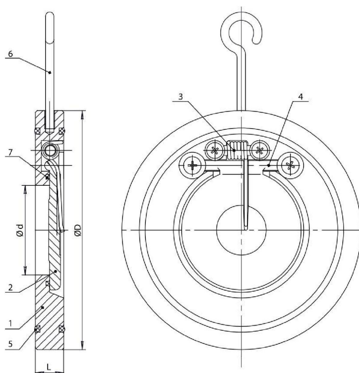
Рисунок 1. Конструкция клапана
