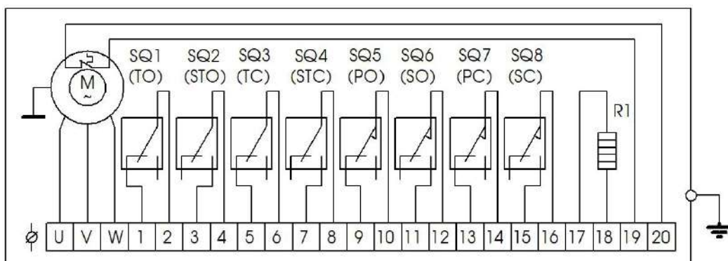
Схема электрическая соединений CE111-41B электропривода неполнооборотного взрывозащищенного исполнения ГЗ-ОФВ типоразмер 8021, 8022, 8023 питанием 3 AC 400В 50Гц
