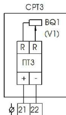
Схема электрическая соединений 802CPT3 с токовым выходом
