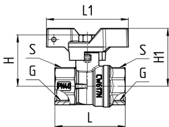
Рисунок 2 – Габаритные размеры крана.
