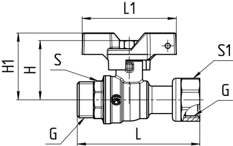
Рисунок 2 – Габаритные размеры крана.
