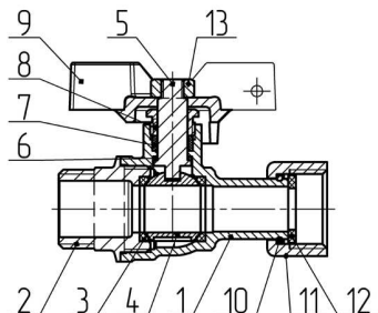
Рисунок 1 – Конструкция шарового крана
