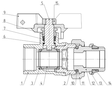
Рисунок 1 – Конструкция шарового крана
