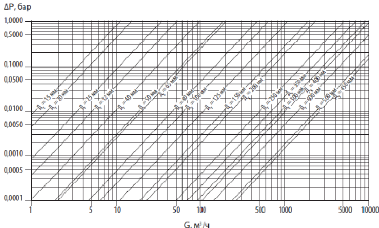
Диаграмма потерь давления крана шарового типа JiP Premium
