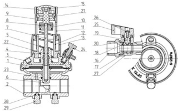
Рисунок 2 – Конструкция клапана
